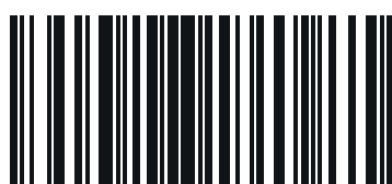
n = 0x03
